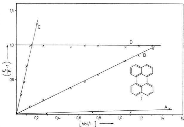
Abb. 1. Stern-Volmer-Geraden für die Fluoreszenzlöschung von Perylen (I) in Toluol bei Raumtemperatur (Anregungswellenlänge 436 nm). Löscher: 1-Chlornaphthalin (Gerade A), 1-Bromnaphthalin (B), 1-Jodnaphthalin (C), Brombenzol (D). Der Übersichtlichkeit halber ist die Gerade D um eine Einheit zu positiven Werten verschoben.
